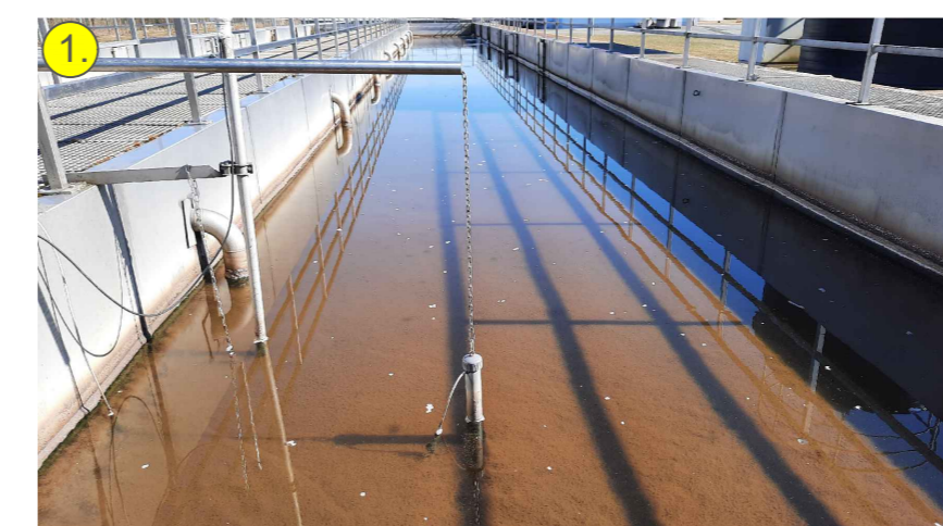
Blick auf Belebungsbecken II mit Sauerstoffmesssonde
